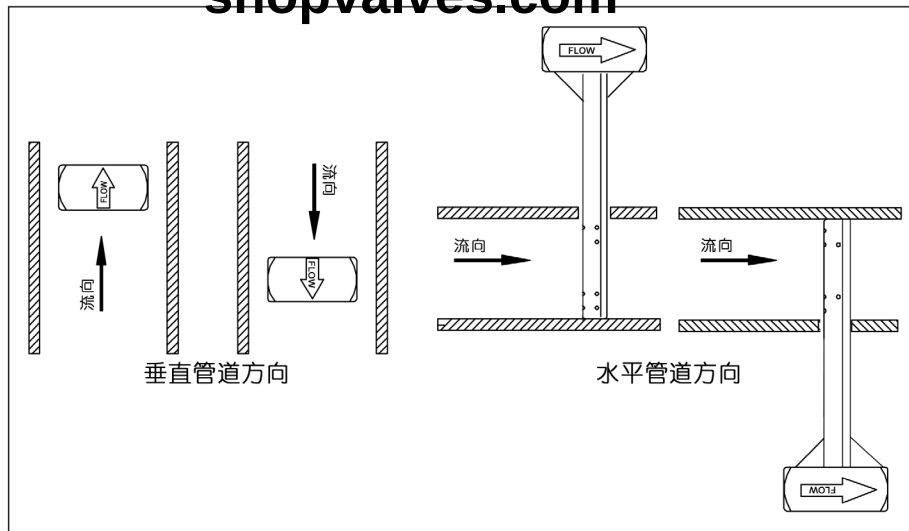
图 4：流体方向
